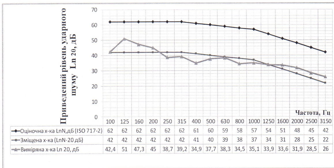
Рисунок 2 – Частотна характеристика приведенного рівня ударного шуму ( L_n 20 , дБ) у звукомірній камері під перекриттям з плаваючою підлогою, укладеною по звукоізоляційному шару із матеріалу A4Sound Floor загальною товщиною 20 мм виробництва ТОВ «ГЛОБАЛ АКУСТИКС»
