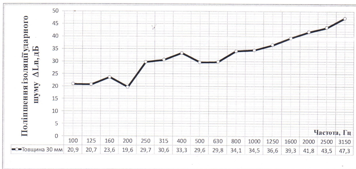
Рисунок 3а – Частотна характеристика поліпшення ізоляції ударного шуму плаваючою підлогою ( \Delta L_{n 30} , дБ) із звукоізоляційним шаром A4Sound Floor загальною товщиною 30 мм виробництва ТОВ «ГЛОБАЛ АКУСТИКС»
