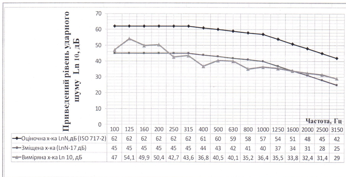
Рисунок 1 – Частотна характеристика приведенного рівня ударного шуму ( L_n 10 , дБ) у звукомірній камері під перекриттям з плаваючою підлогою, укладеною по звукоізоляційному шару із матеріалу A4Sound Floor товщиною 10 мм виробництва ТОВ «ГЛОБАЛ АКУСТИКС»
