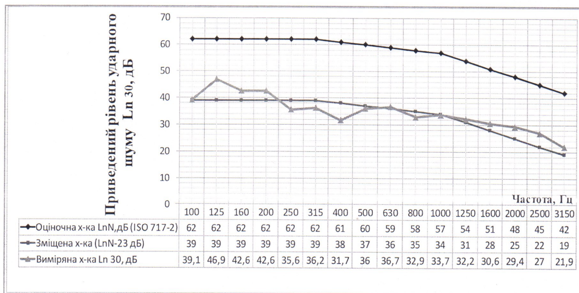
Рисунок 3 – Частотна характеристика приведенного рівня ударного шуму ( L_{n 30} , дБ) у звукомірній камері під перекриттям з плаваючою підлогою, укладеною по звукоізоляційному шару із матеріалу A4Sound Floor загальною товщиною 30 мм виробництва ТОВ «ГЛОБАЛ АКУСТИКС»
