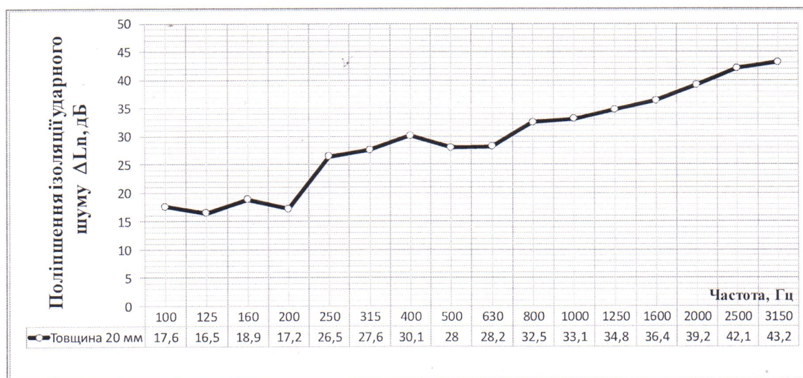
Рисунок 2а – Частотна характеристика поліпшення ізоляції ударного шуму плаваючою підлогою ( \Delta L_n 20 , дБ) із звукоізоляційним шаром A4Sound Floor загальною товщиною 20 мм виробництва ТОВ «ГЛОБАЛ АКУСТИКС»
