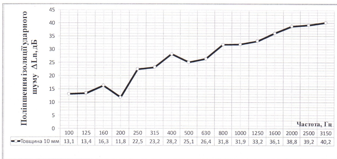
Рисунок 1а – Частотна характеристика поліпшення ізоляції ударного шуму плаваючою підлогою ( \Delta L_n 10 , дБ) із звукоізоляційним шаром A4Sound Floor товщиною 10 мм виробництва ТОВ «ГЛОБАЛ АКУСТИКС»
